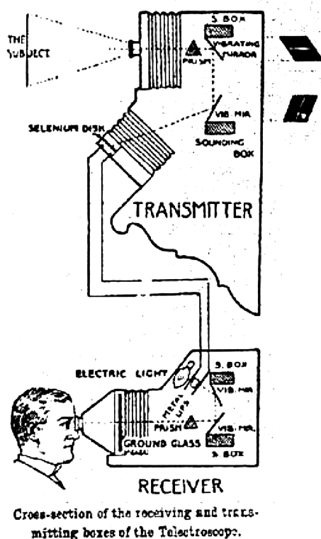
Obr. 2. Schéma Szczepanikova telectroskopu otištěné v článku C. Moffetta „Seeing by wire“ (Přenos obrazu pomocí vodiče) v časopisu Pearson's Magazine, 1899, s. 490–496.
